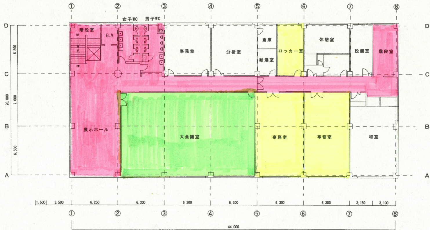
管理棟 3階平面図 S=1/200
