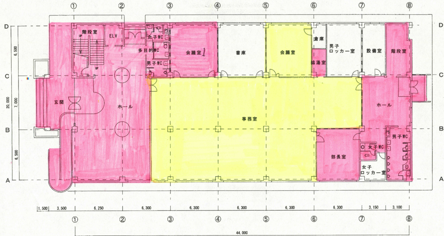
管理棟 1階平面図 S=1/200
