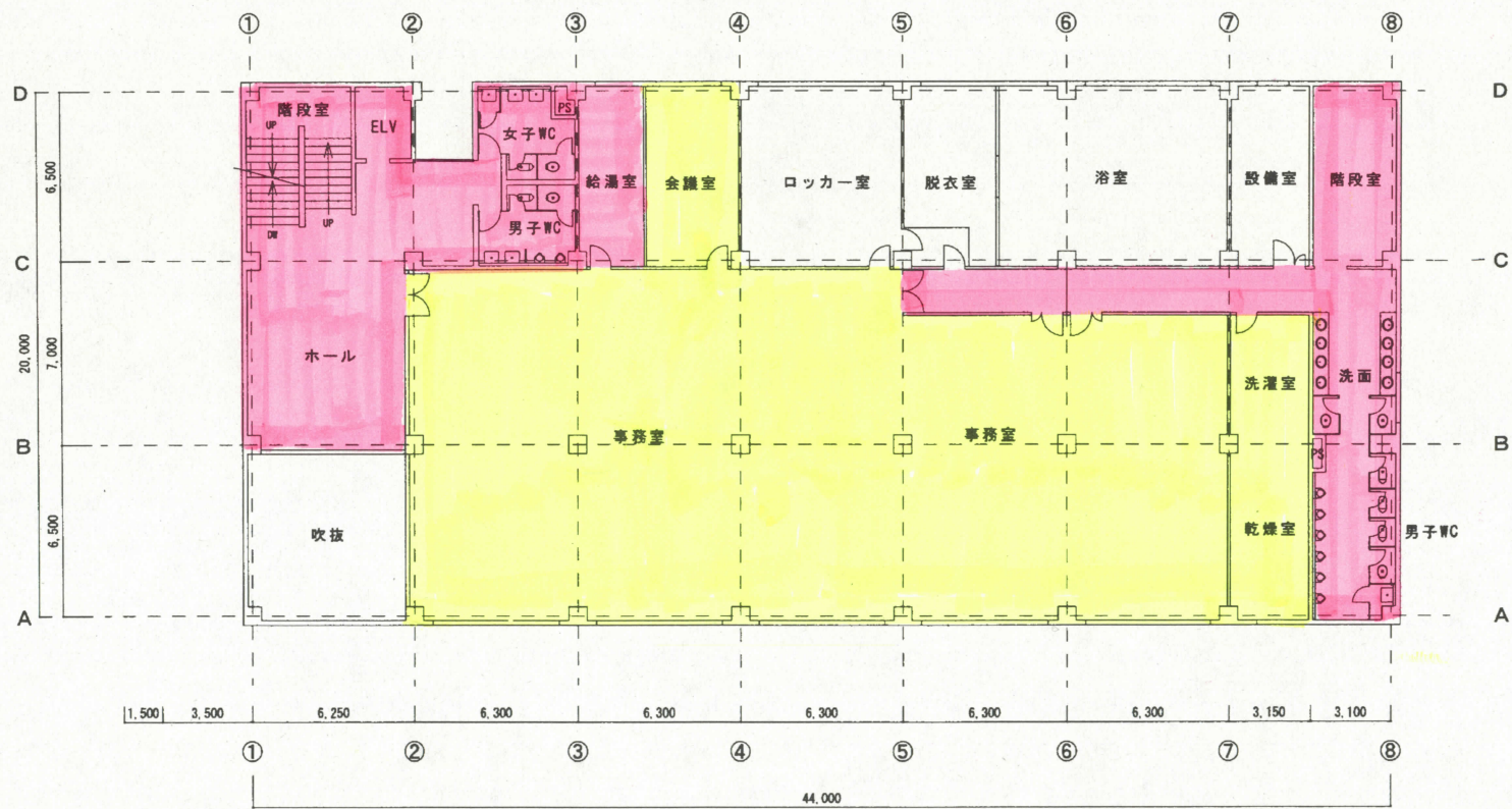
管理棟 2階平面図 1/200
